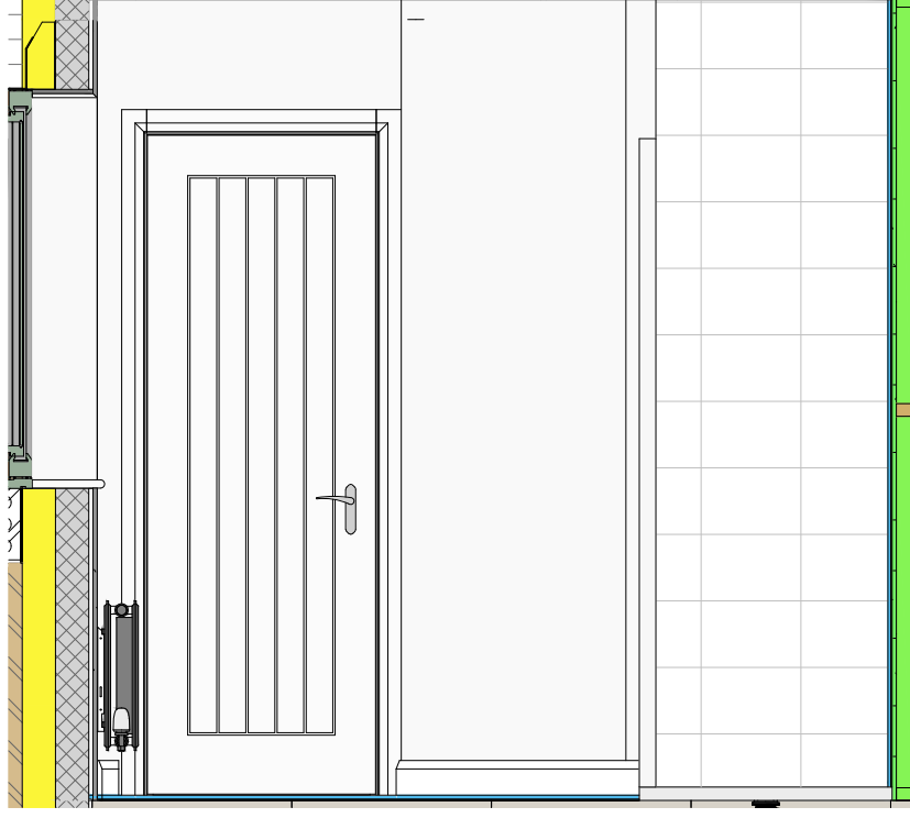
D Ensuite - View D 1 : 25
