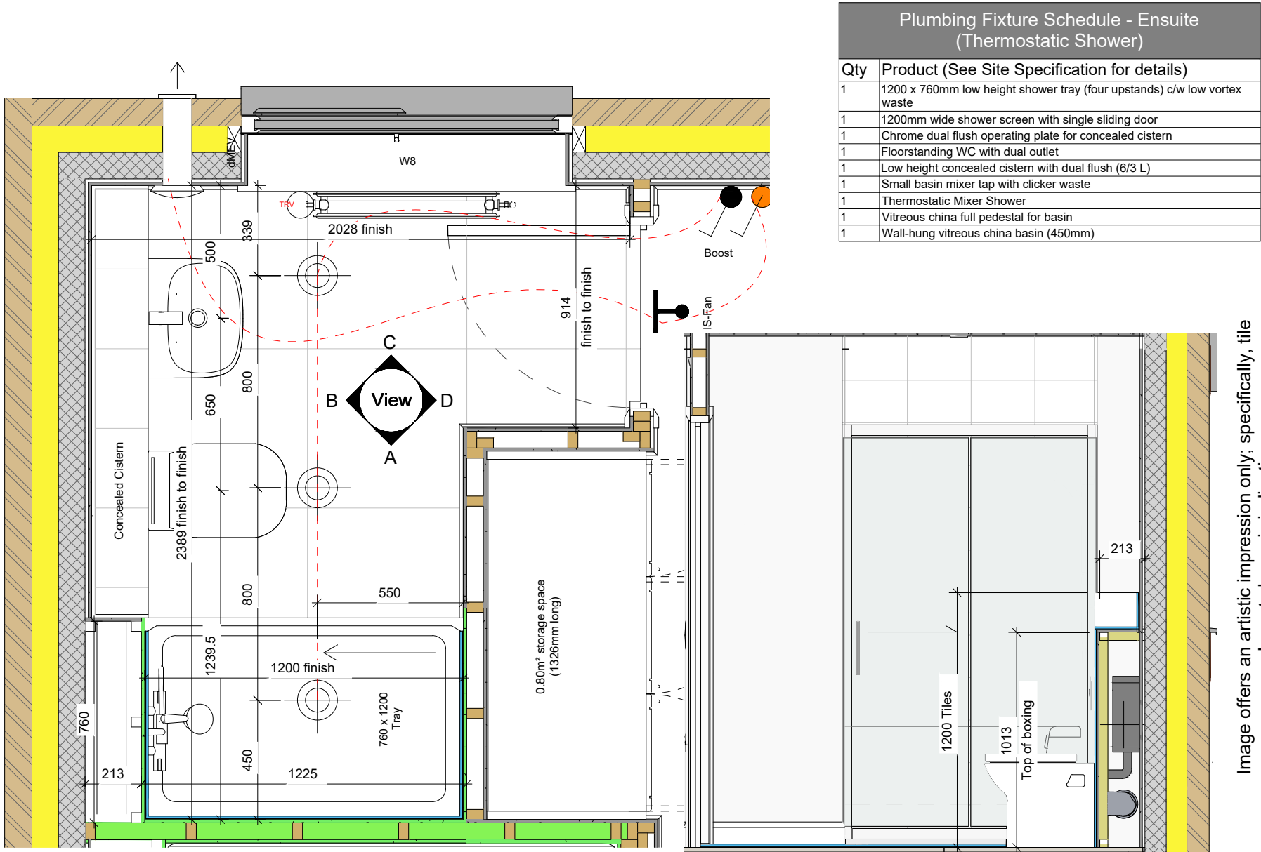
1 Ensuite Layout 1 : 20
