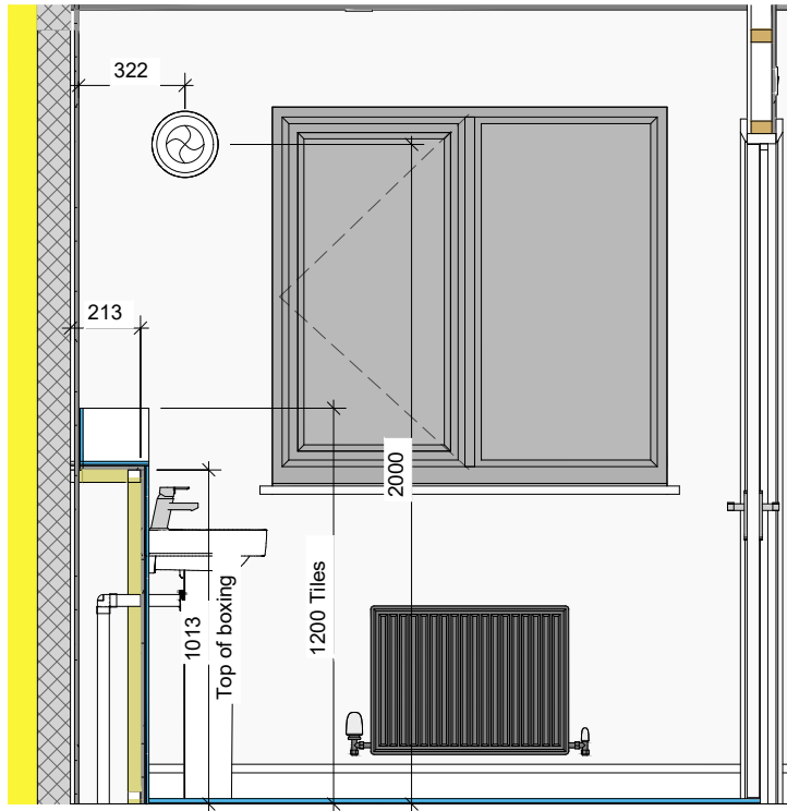
A Ensuite - View A 1 : 25
