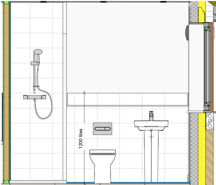
1 Ensuite Layout 1 : 20
